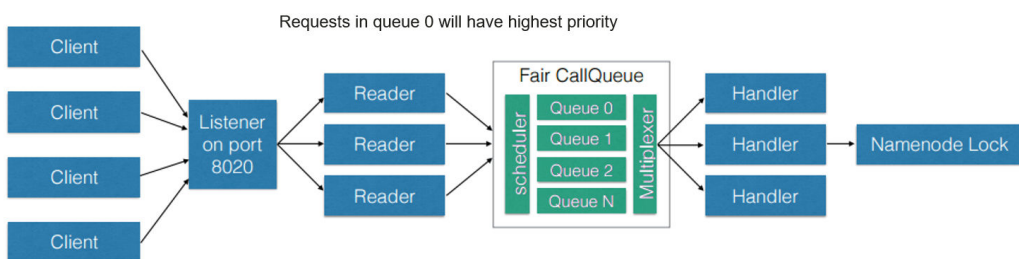
图 8-5 基于 FAIRCallQueue 的 NameNode 请求处理
