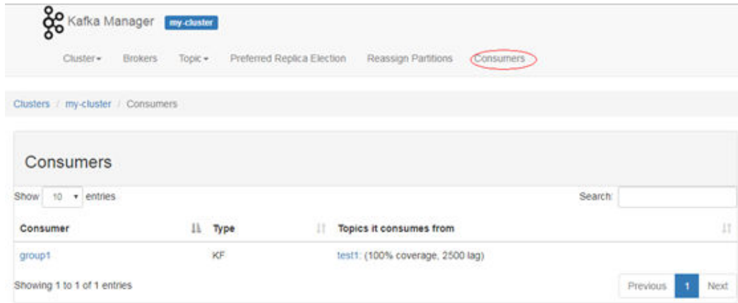
图 15-9 Consumers 列表
