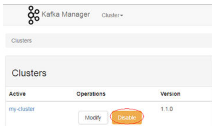
图 15-3 停用集群
