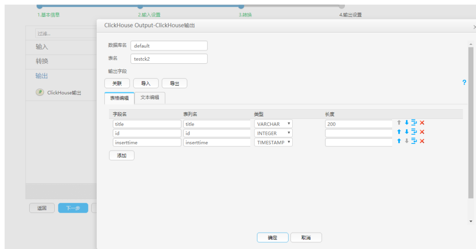
图 16-39 算子输出
