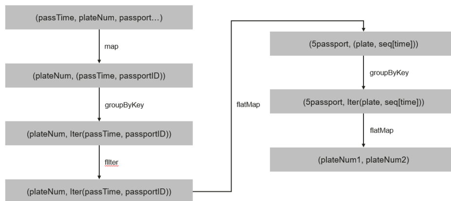
图 24-7 实现 2 逻辑
