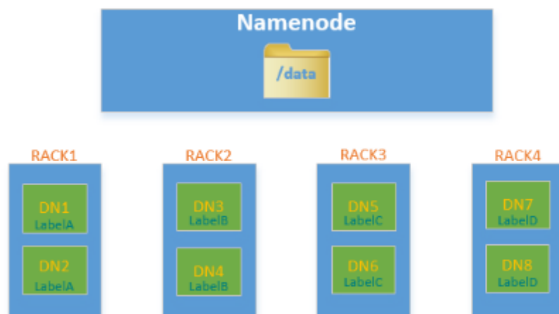
图 8-7 场景样例
