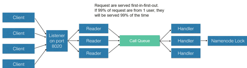
图 8-4 基于 FIFO 调用队列的 NameNode 请求处理
