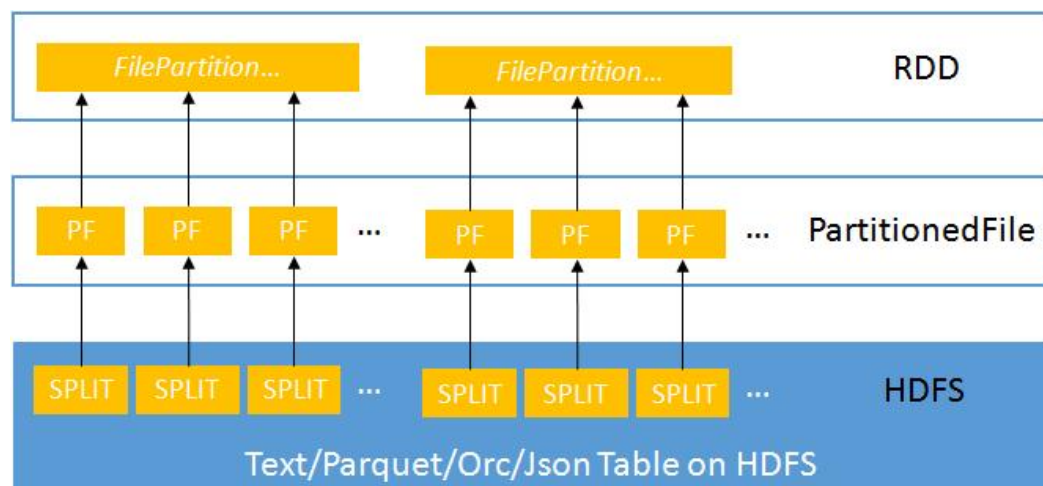
图 24-8 小文件合并
