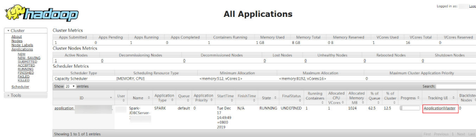
图 23-5 ApplicationMaster
