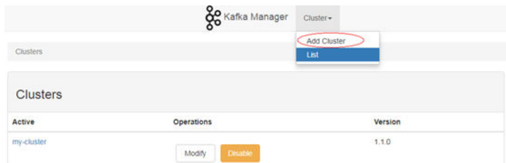
图 15-1 添加集群
