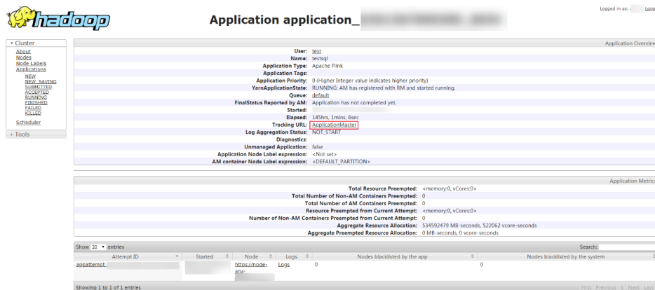
图 5-4 application
