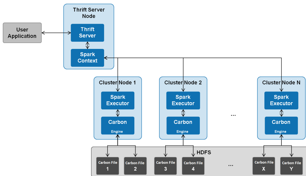
图 2-2 CarbonData 结构
